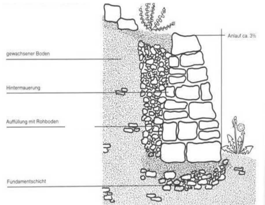
Abbildung 20: Exemplarische Darstellung zum Bau einer Trockenmauer
