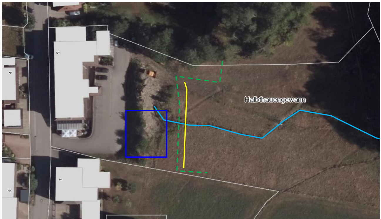
Abbildung 12: Vom Feuersalamander besiedelter Graben (hellblau), geplantes Baufenster (dunkelblau), neuer Grabenabschnitt (gelb), amphibiensicherer Schutzzaun (grün gestrichelt) (Quelle Luftbild: LUBW)
