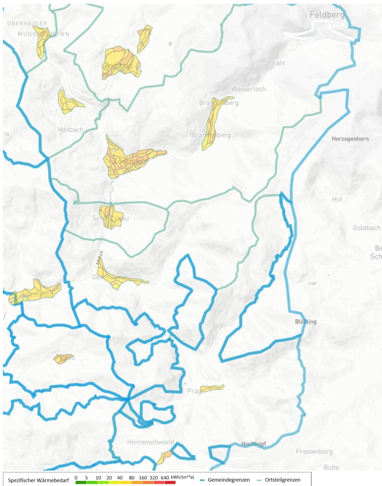
Abbildung 19: Gebiete nach spezifischem Wärmebedarf in Todtnau.
