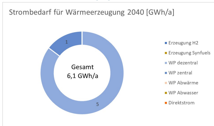
Abbildung 17: Strombedarf für Wärmeerzeugung 2040 in Todtnau.
