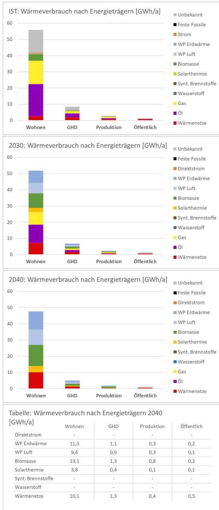
Abbildung 16: Wärmebedarf nach Energieträgern und nach Sektoren in Todtnau für den IST-Zustand, sowie für das Zwischen-szenario 2030 und für das Zielszenario 2040.
