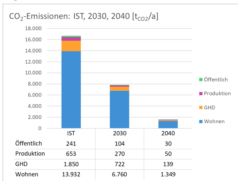
Abbildung 18: CO 2 -Bilanzen für 2020, 2030 und 2040 für Todtnau.
