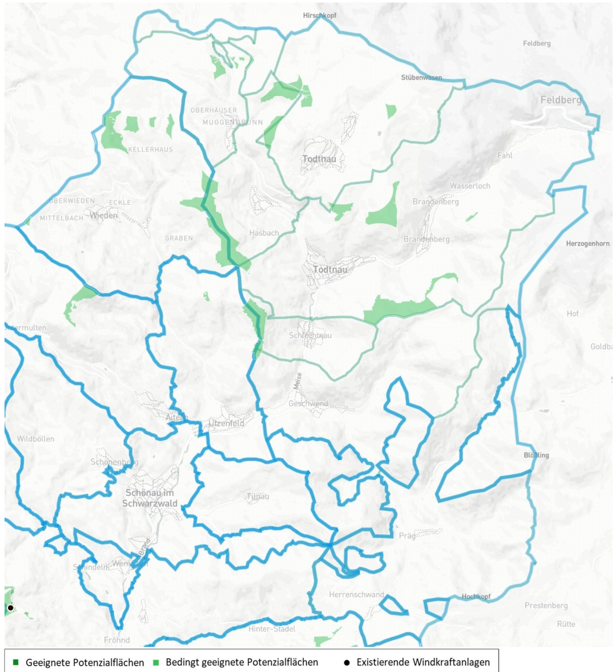
Abbildung 11: Geeignete und bedingt geeignete Windpotenzialflächen sowie bereits existierende Windenergieanlagen.
