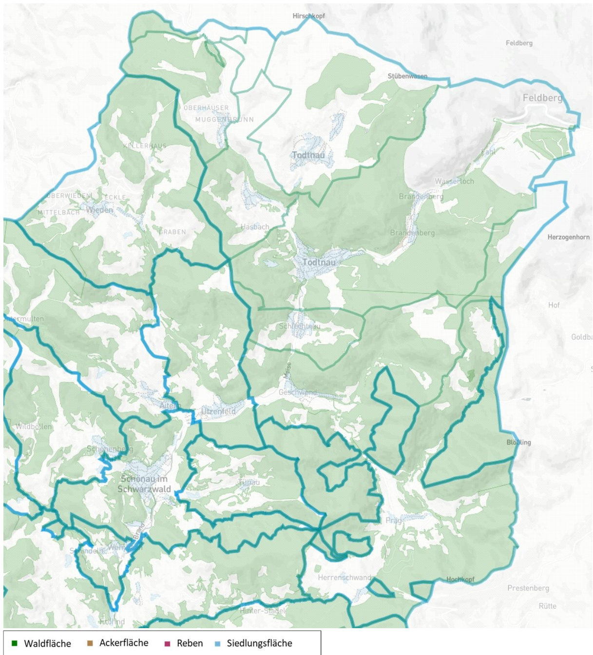
Abbildung 12: Biomasse-Potenzialflächen in Todtnau.
