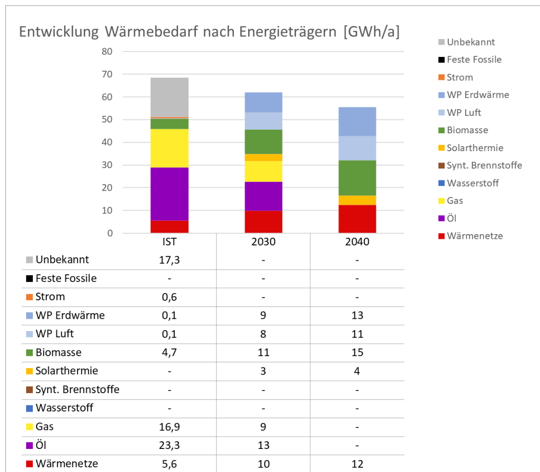
Abbildung 14: Entwicklung des Wärmebedarfs und eingesetzte Energieträger in Todtnau: IST, 2030, 2040. Die angesetzten Reduktionsfaktoren sind im vorigen Kapitel erläutert.
