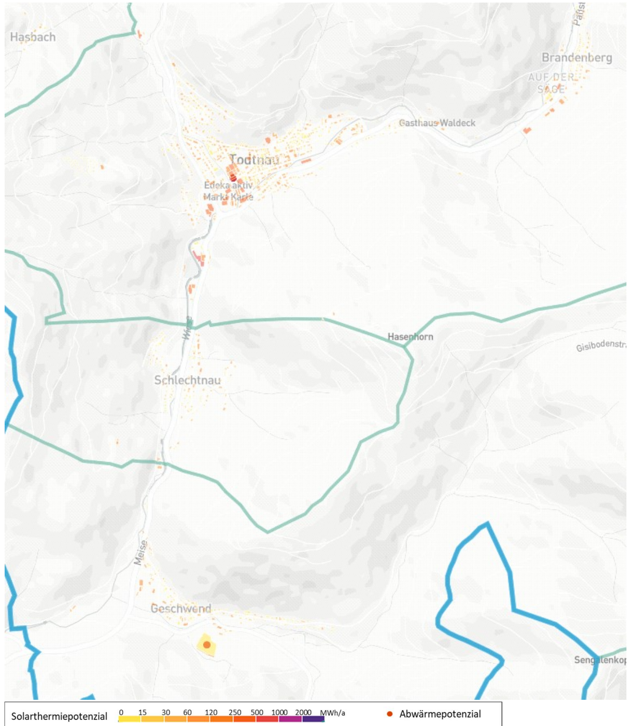
Abbildung 10: Innerörtliche Potenziale: Solarthermie und industrielle Abwärme in Todtnau. (Die PV-Potenziale nutzen die identischen Flächen.) Zur besseren Erkennbarkeit ist ggf. nur ein Ausschnitt dargestellt.
