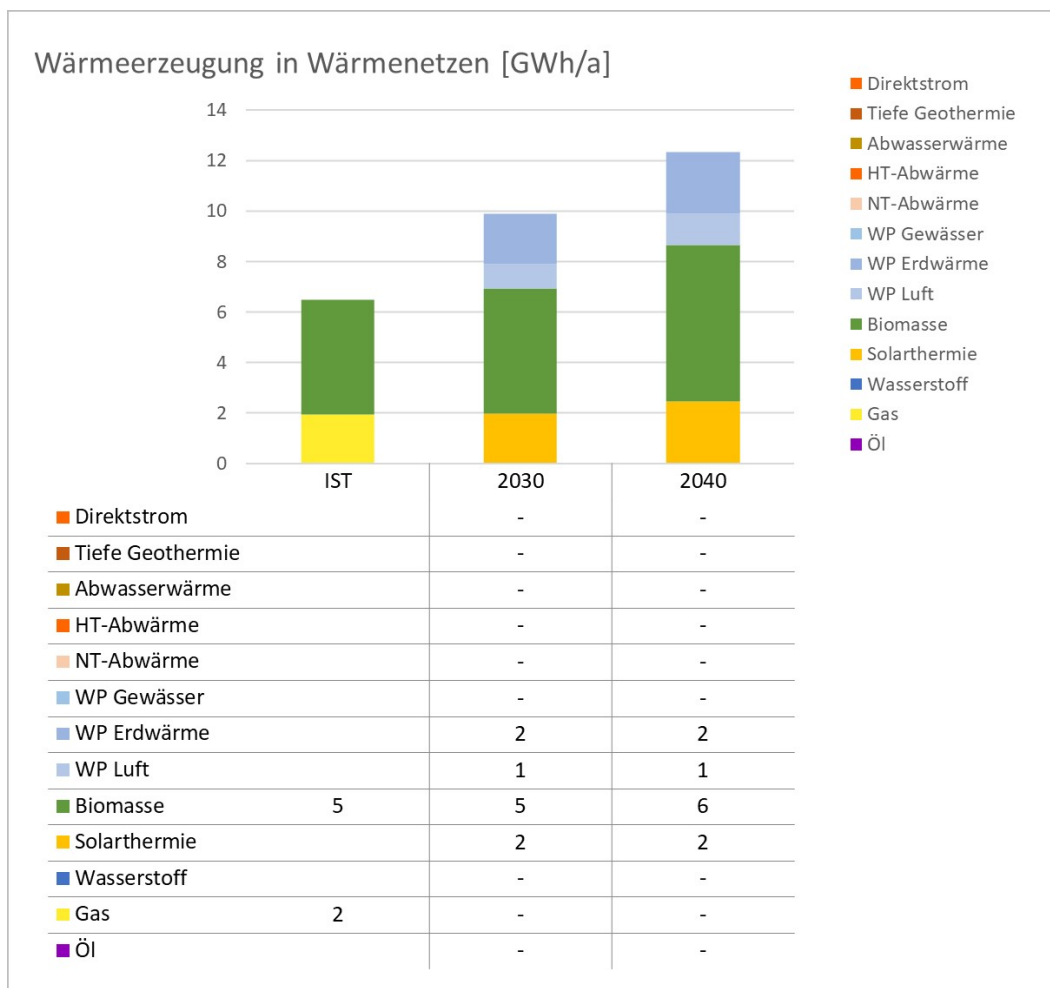
Abbildung 15: Eingesetzte Energieträger zur Wärmeversorgung der Wärmenetze in Todtnau: IST, 2030, 2040.
