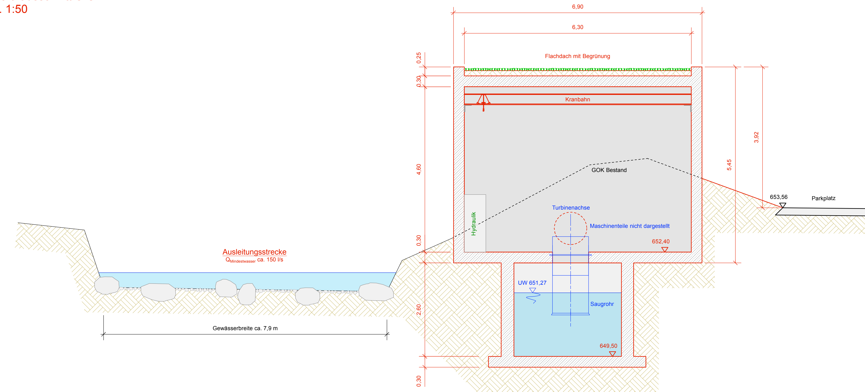
Krafthauschnitt C-C M. 1:50
