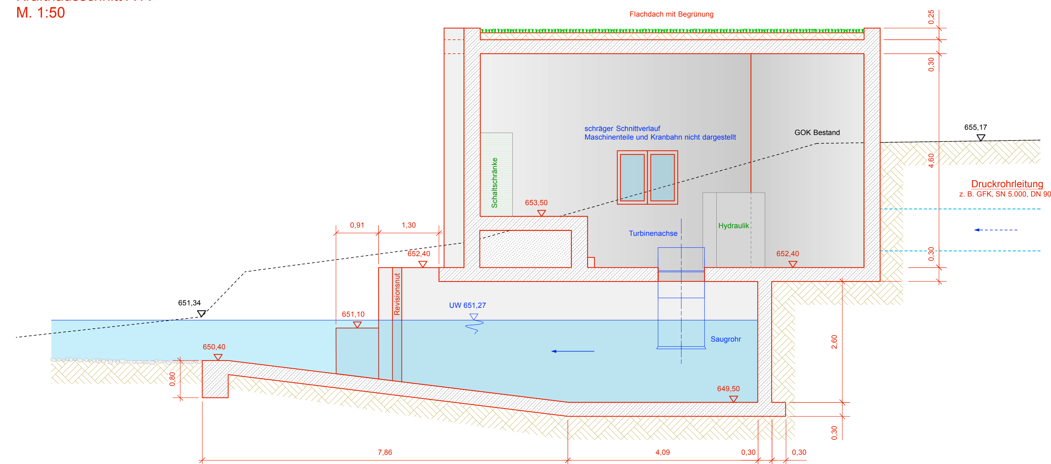
Krafthauschnitt A-A M. 1:50
