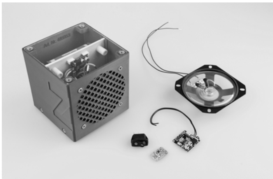
ZAHORANSKY-Lautsprecher-Azubi-Projekt 2022
